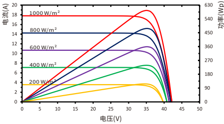
RSM110-8-595BHDG 不同辐照度下, I-V 曲线图
