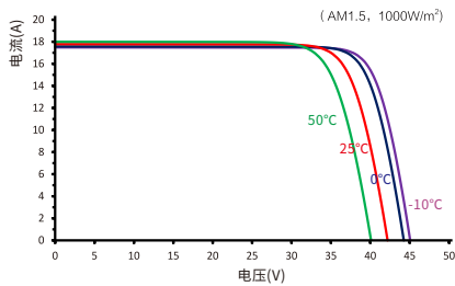
不同电池温度下, I-V 曲线图
